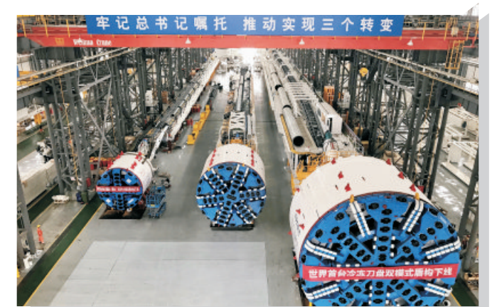
中铁华隧盾构机生产车间
